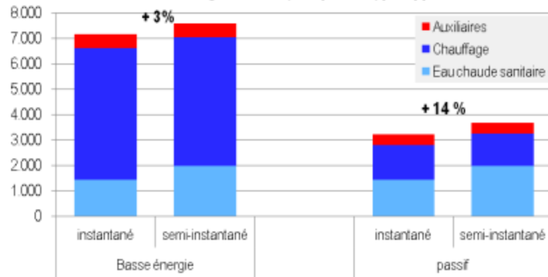
Consommation d'énergie annuelle (kWh primaire) par appartement
